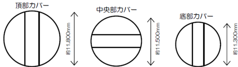
シールドプラグ 各カバーの寸法
