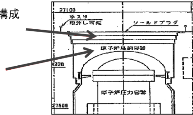
シールドプラグ断面図
